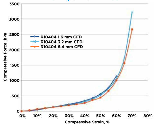
CFD per ASTM D1667
